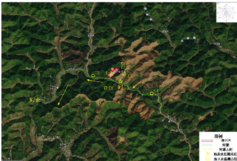
图 5.2-4 地表水及地下水监测布点图
