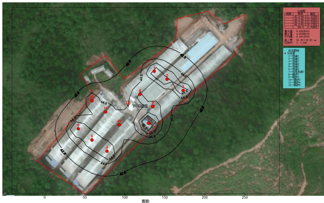
图 6.4-2 建设项目等声值线图
