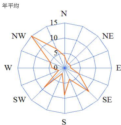
图 6.1-1 兴宁市风向玫瑰图
