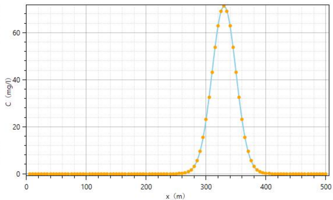
图 6.3-2（2）储罐破损渗漏 1000 天石油类污染物不同距离浓度预测曲线
