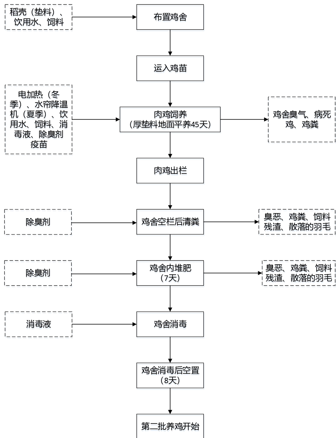
图 3.2-1 原有项目养殖工艺流程及产污环节
