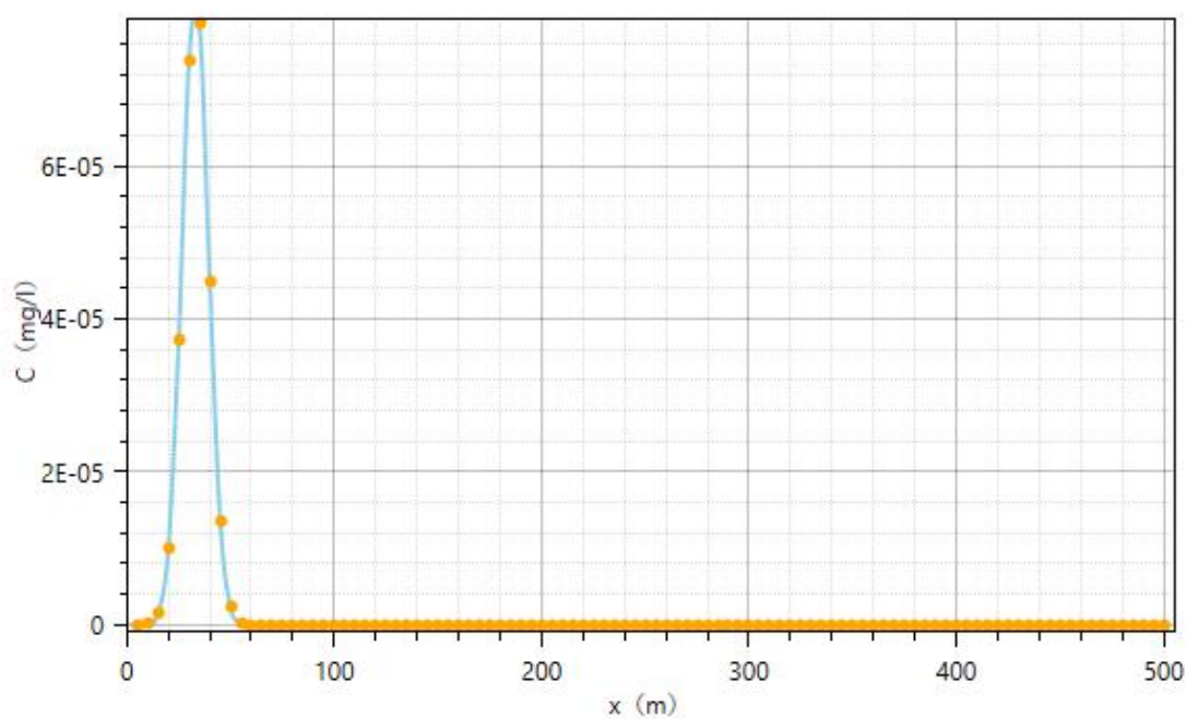
图 6.3-3 (3) 化粪池污水池及污水管道破裂 100 天氨氮不同距离浓度预测曲线
