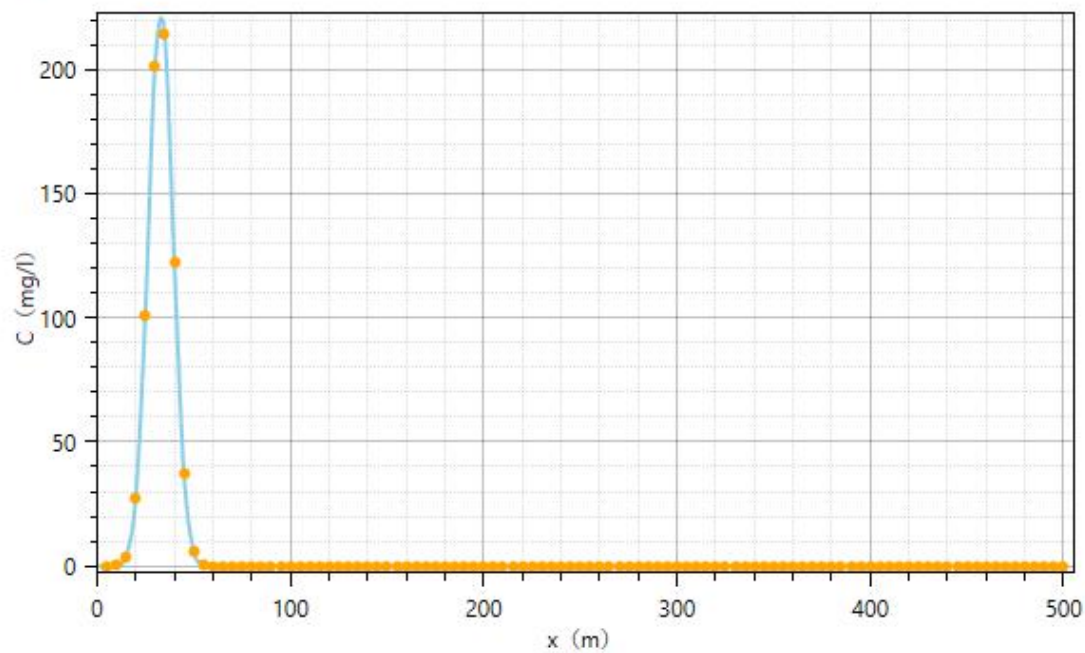
图 6.3-2（1）柴油储罐破损渗漏 100 天石油类污染物不同距离浓度预测曲线
