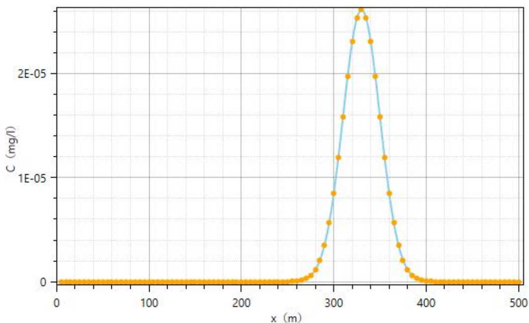
图 6.3-3 (4) 化粪池污水池及污水管道破裂 1000 天氨氮不同距离浓度预测曲线
