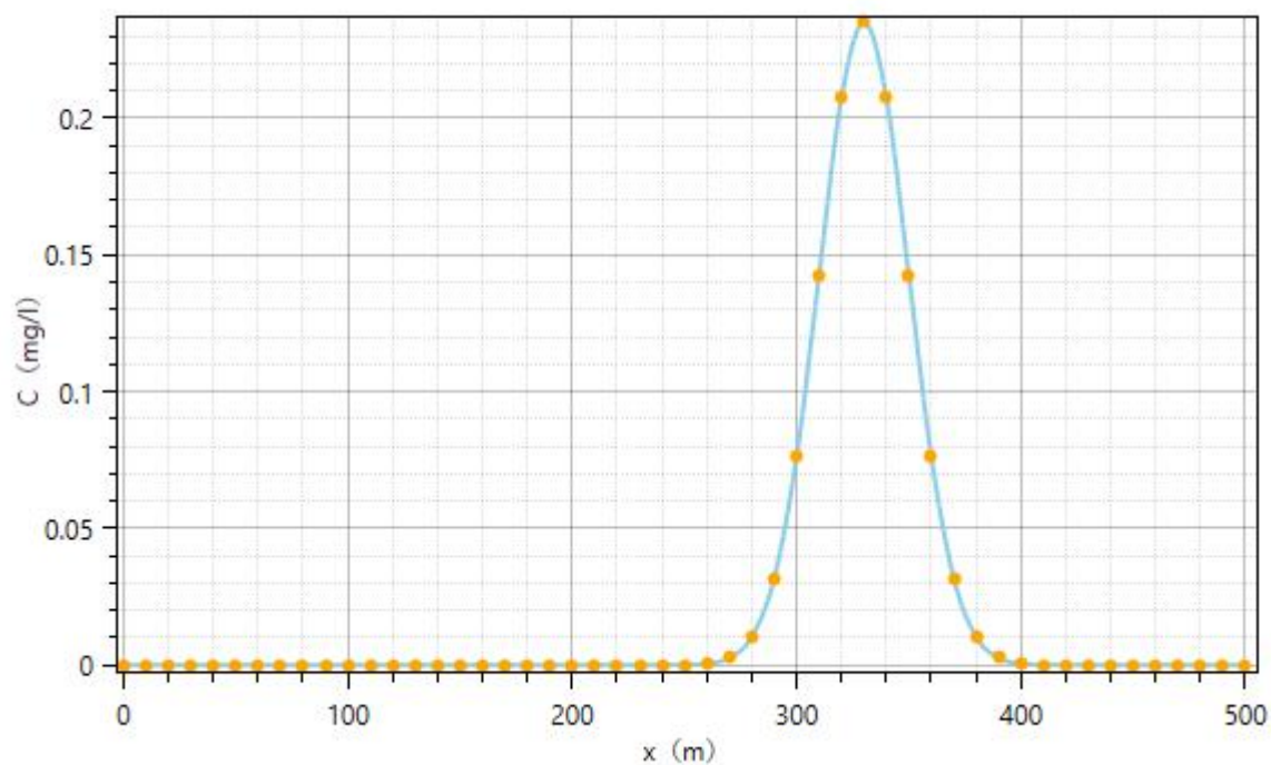
图 6.3-3 (2) 化粪池污水池及污水管道破裂 1000 天 COD 不同距离浓度预测曲线
