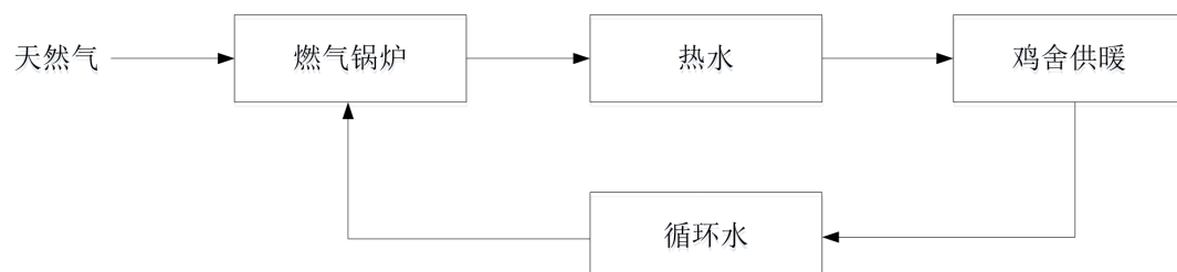
图 4.1-2 供热系统流程示意图
