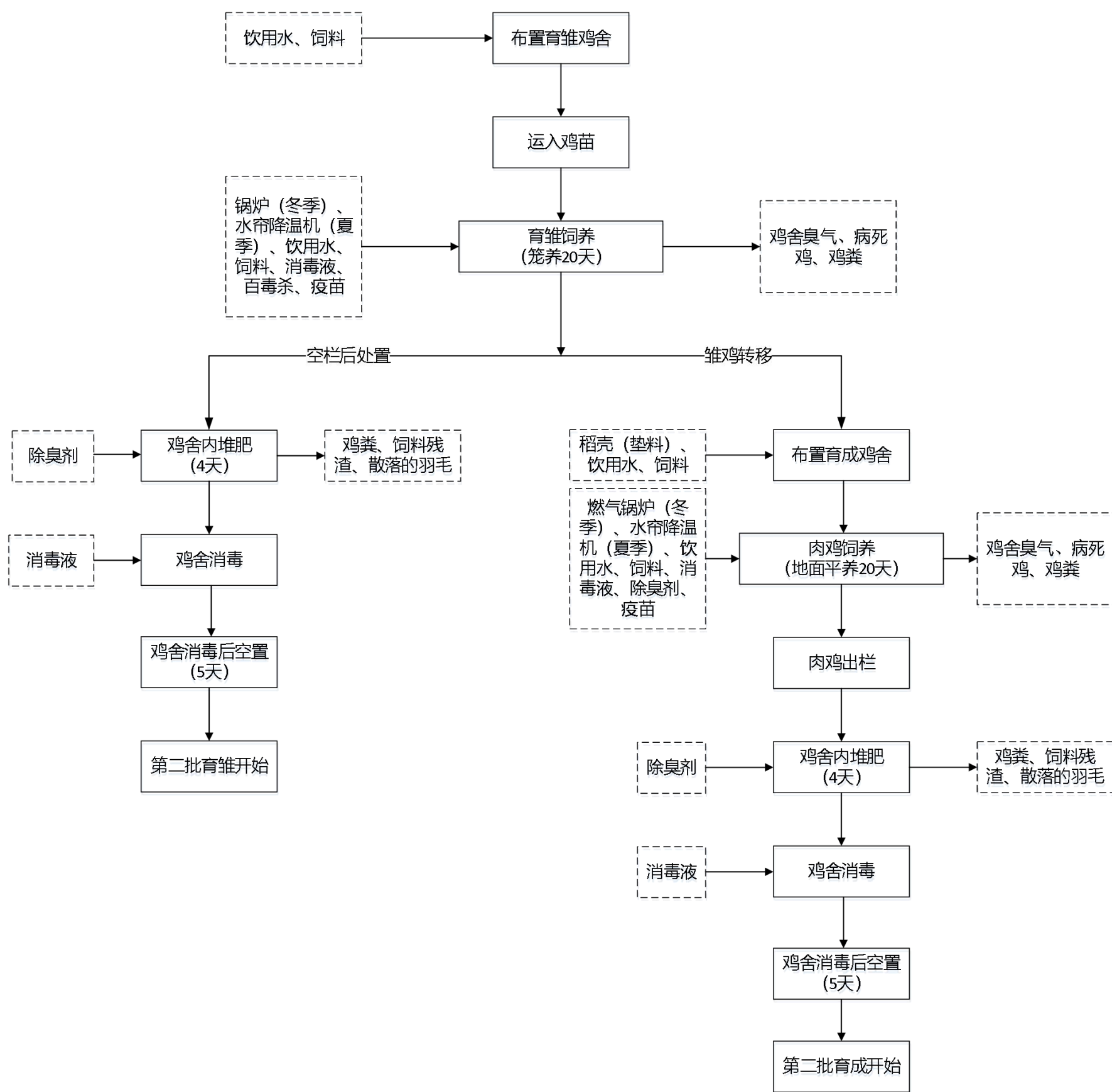
图 4.3-1 本项目生产工艺流程及排污节点示意图
