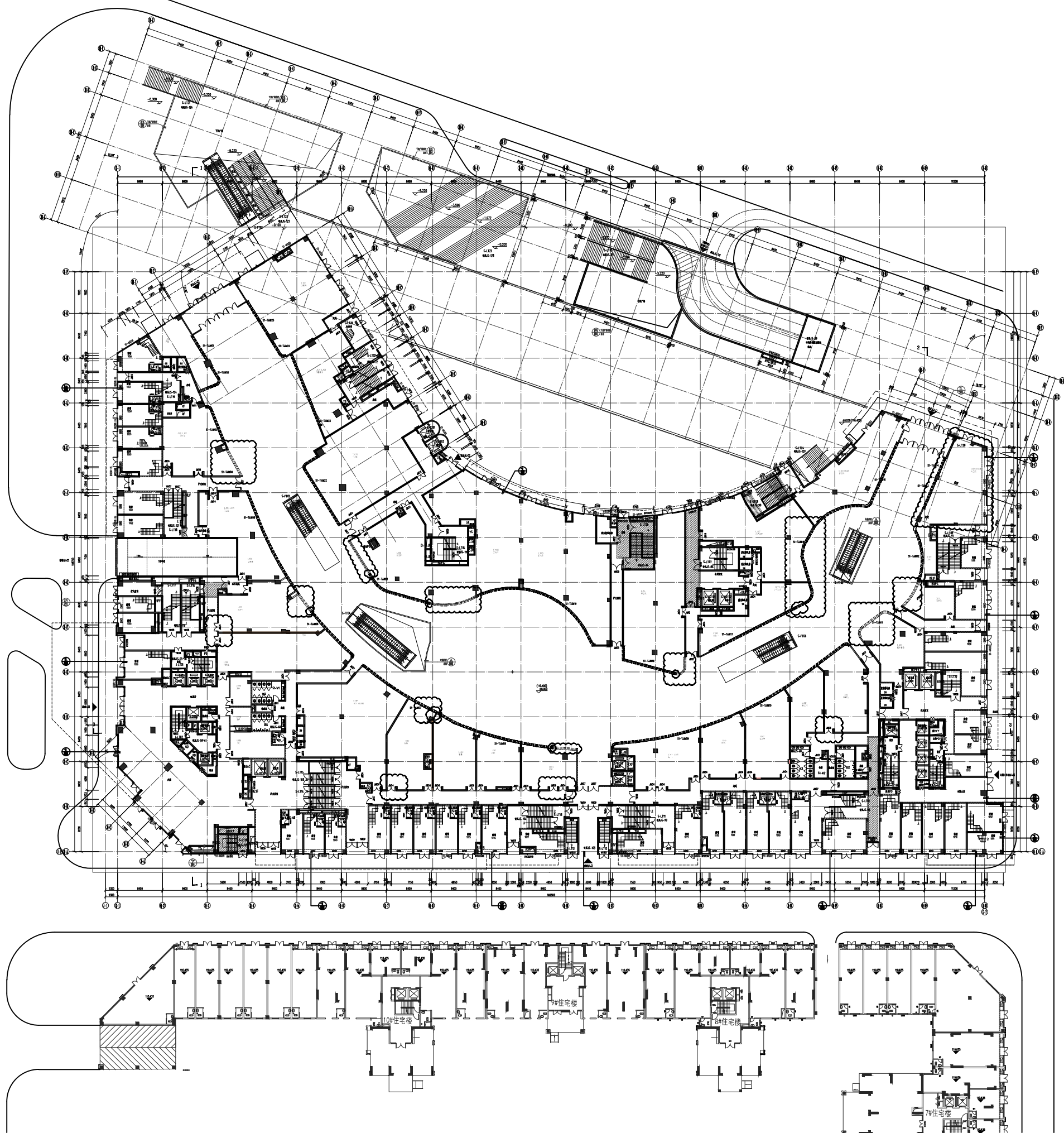
一层平面图
