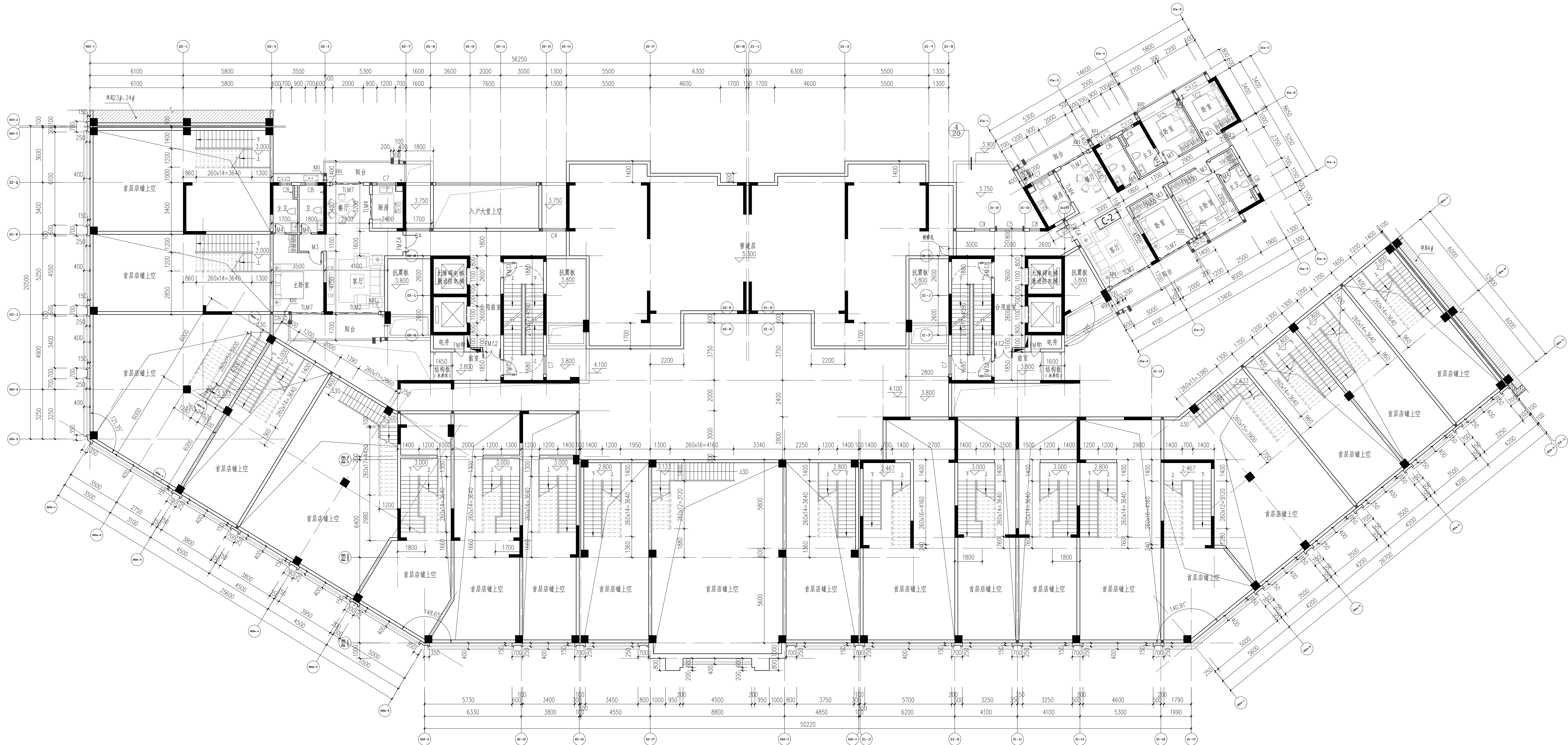
二层平面图 1:100
