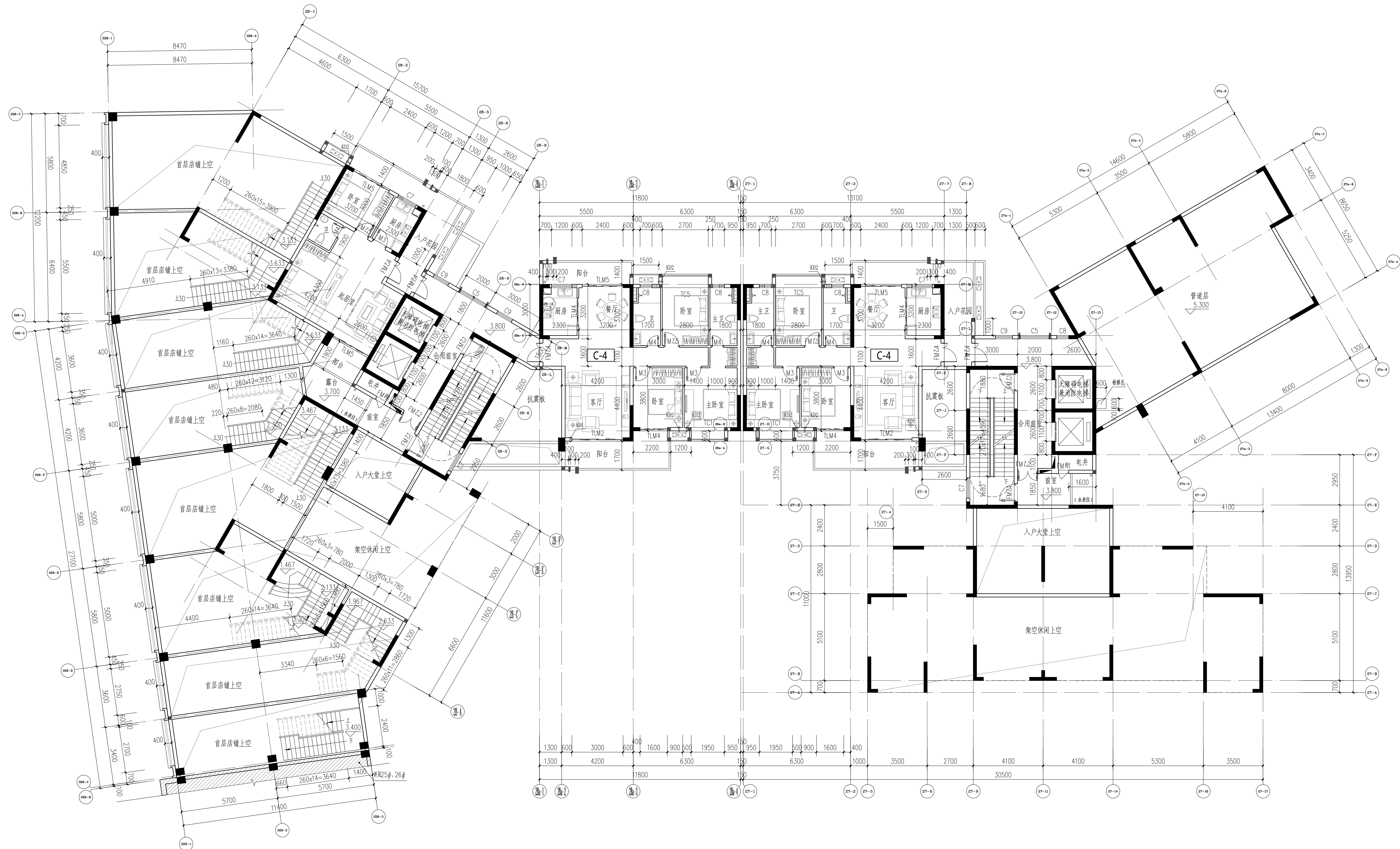
二层平面图 1:100
