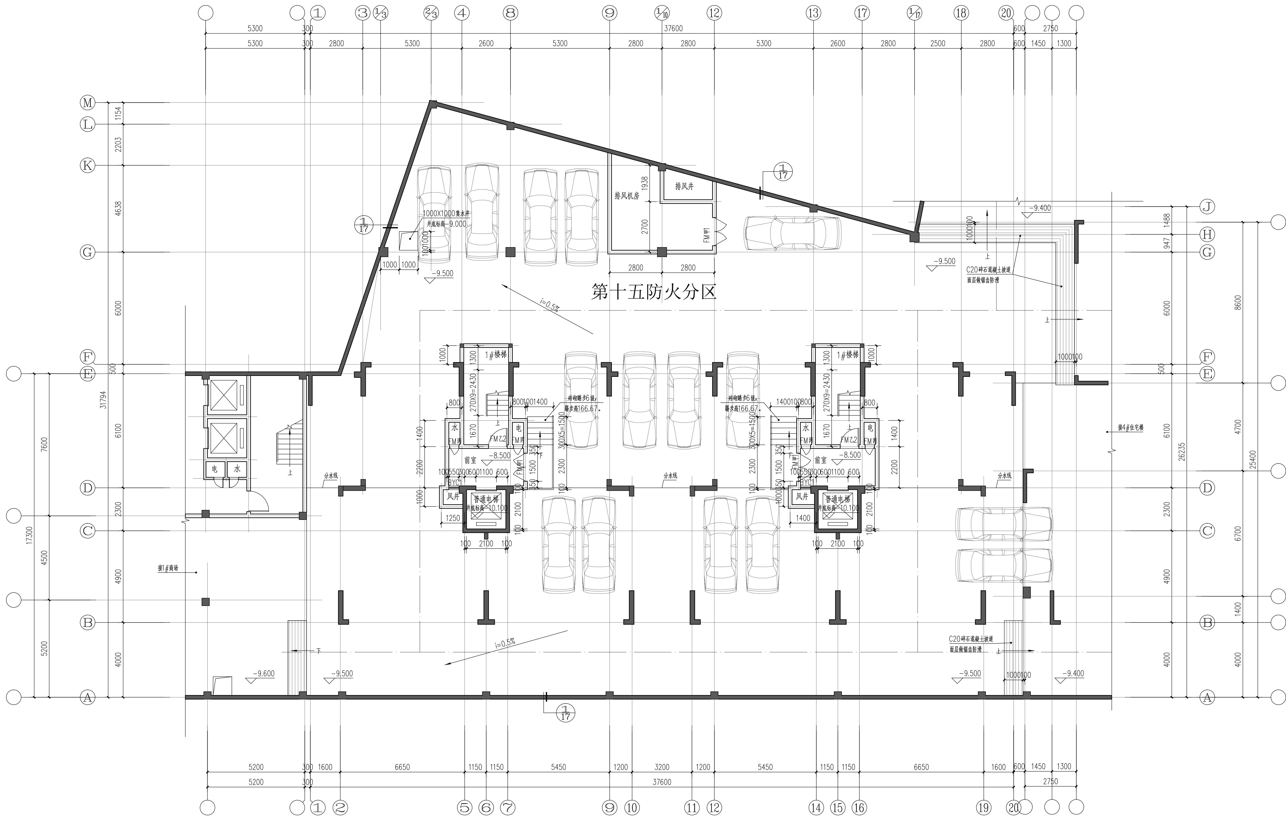
地下二层平面图 1:100
