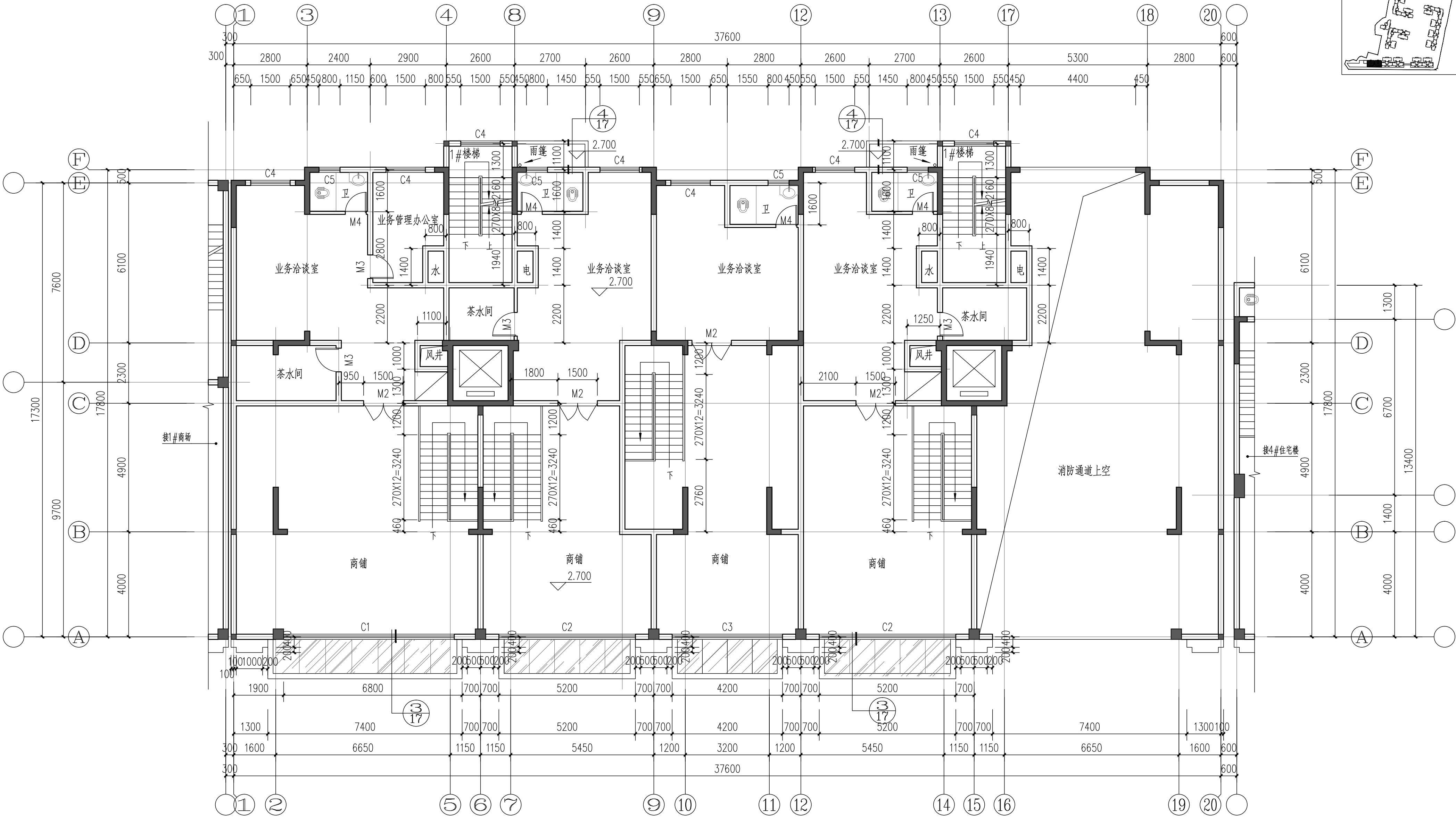
二层平面图 1:100
