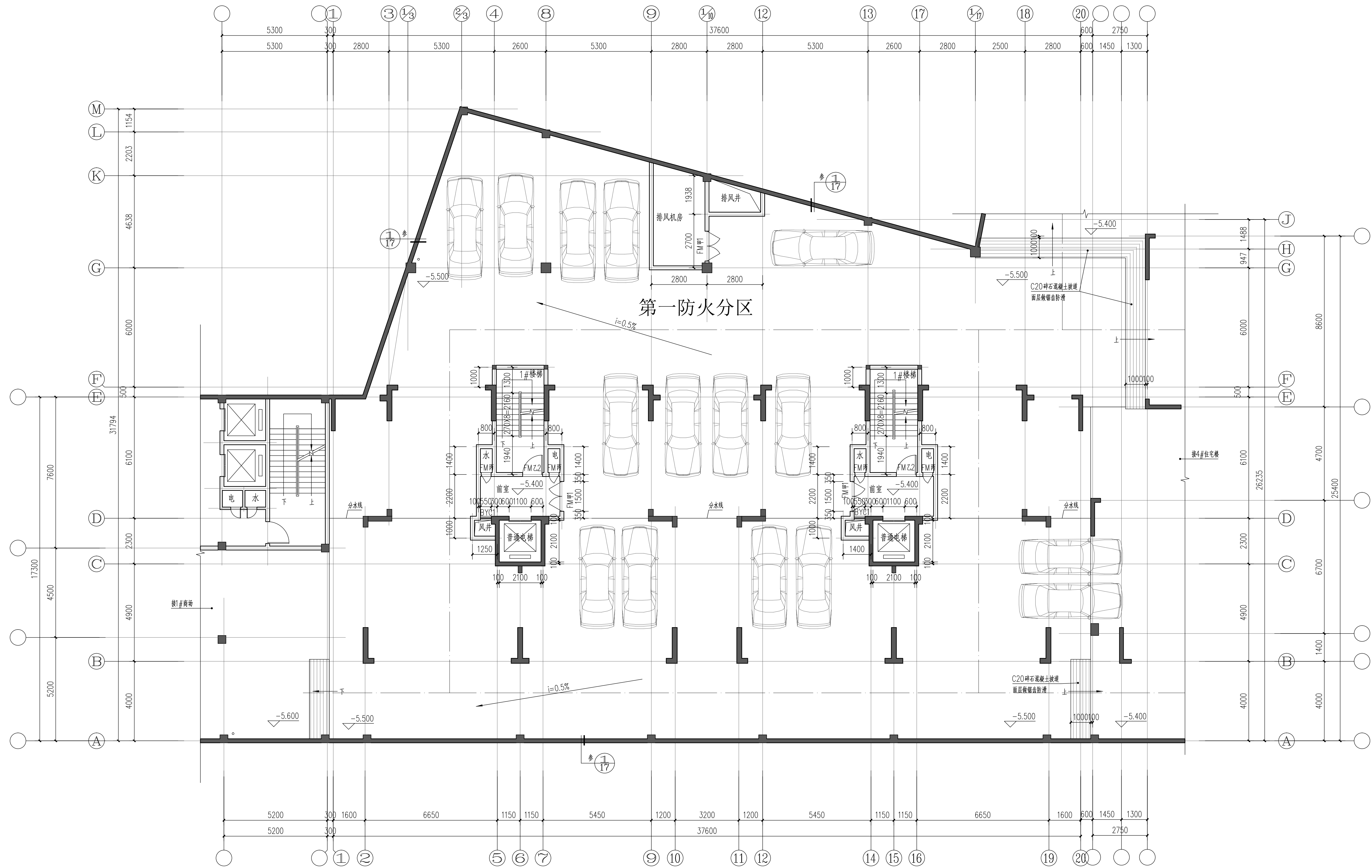
地下一层平面图 1:100
