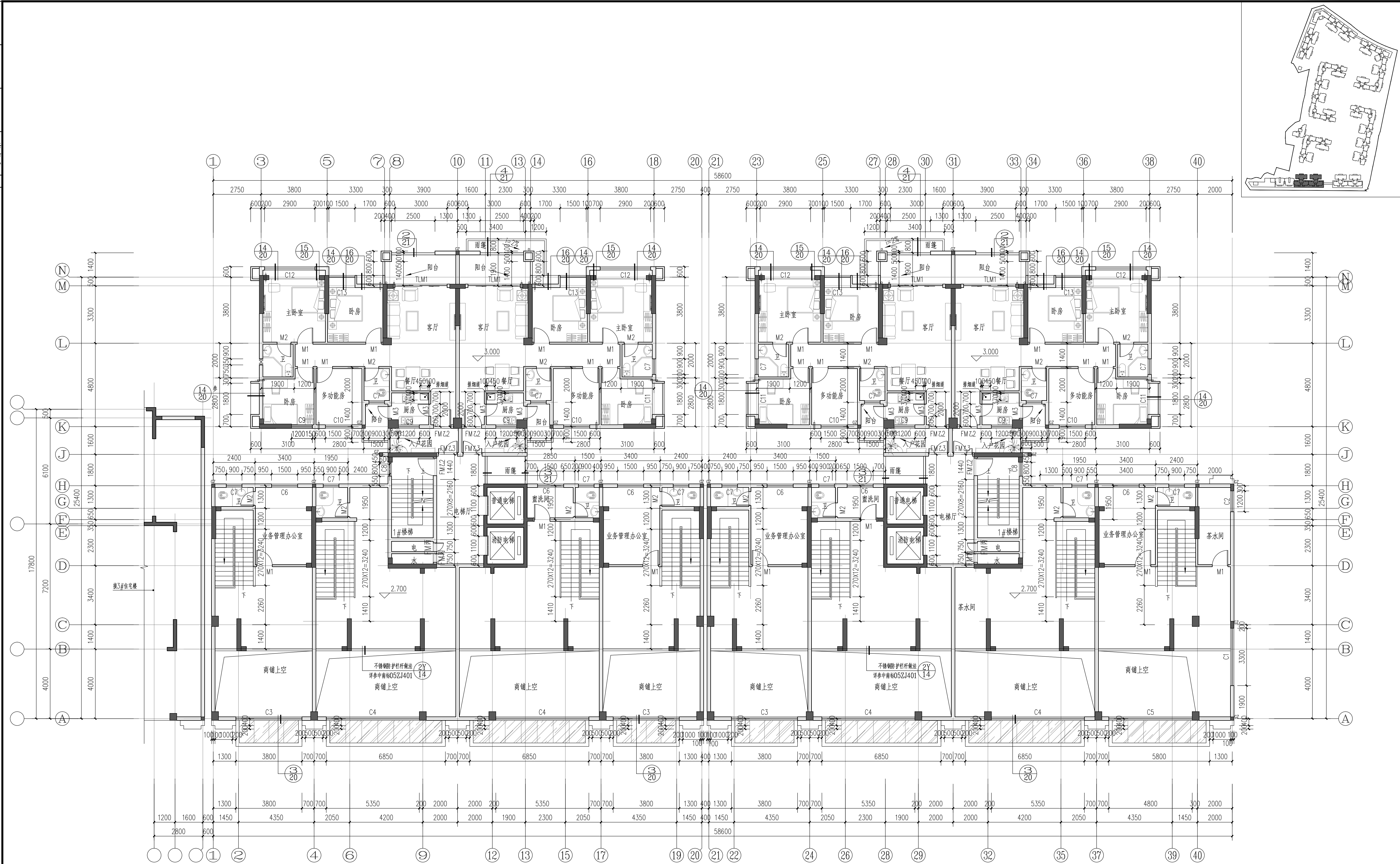
二层平面图 1:100
