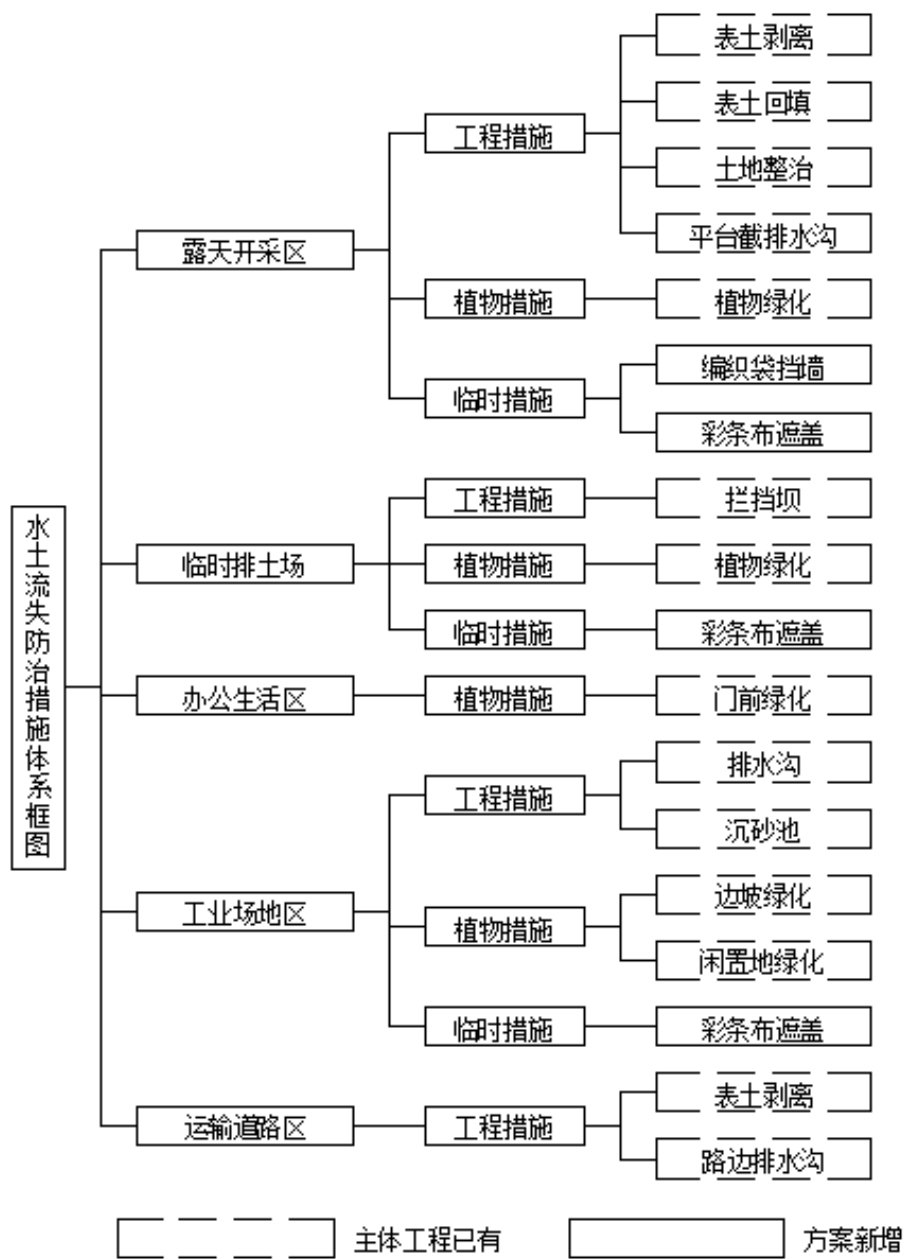
图 5-1 水土流失防治体系框
