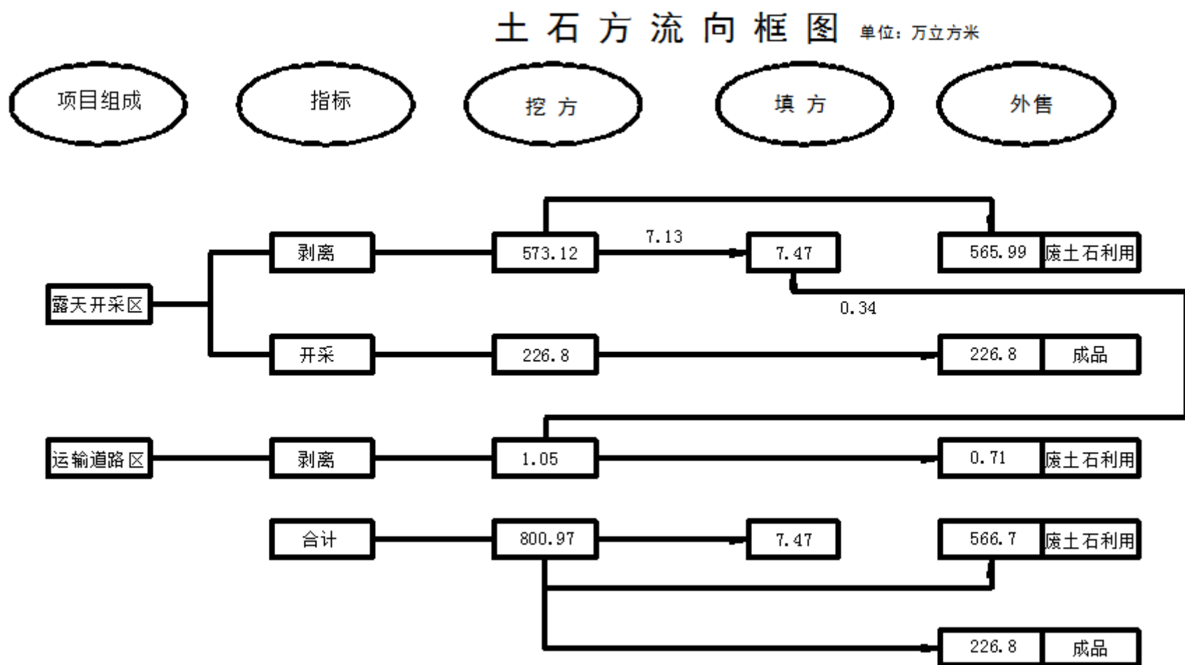
图 2-2 土石方流向图
