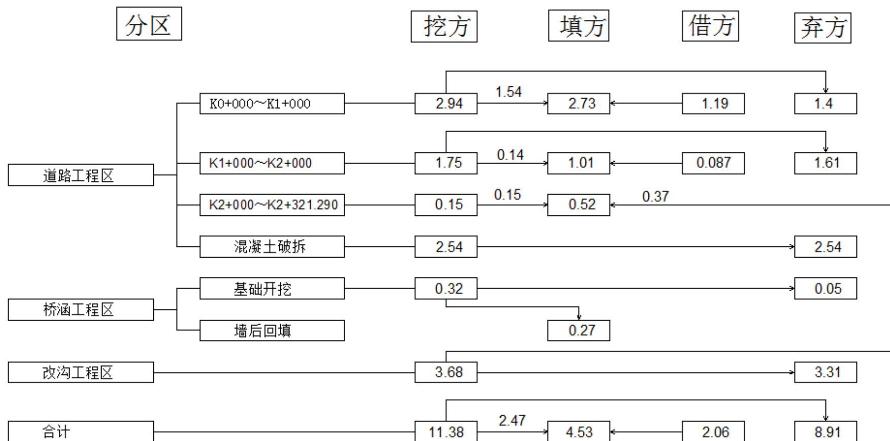
图2-3 土石方流向图单位：万 \text{m}^3
