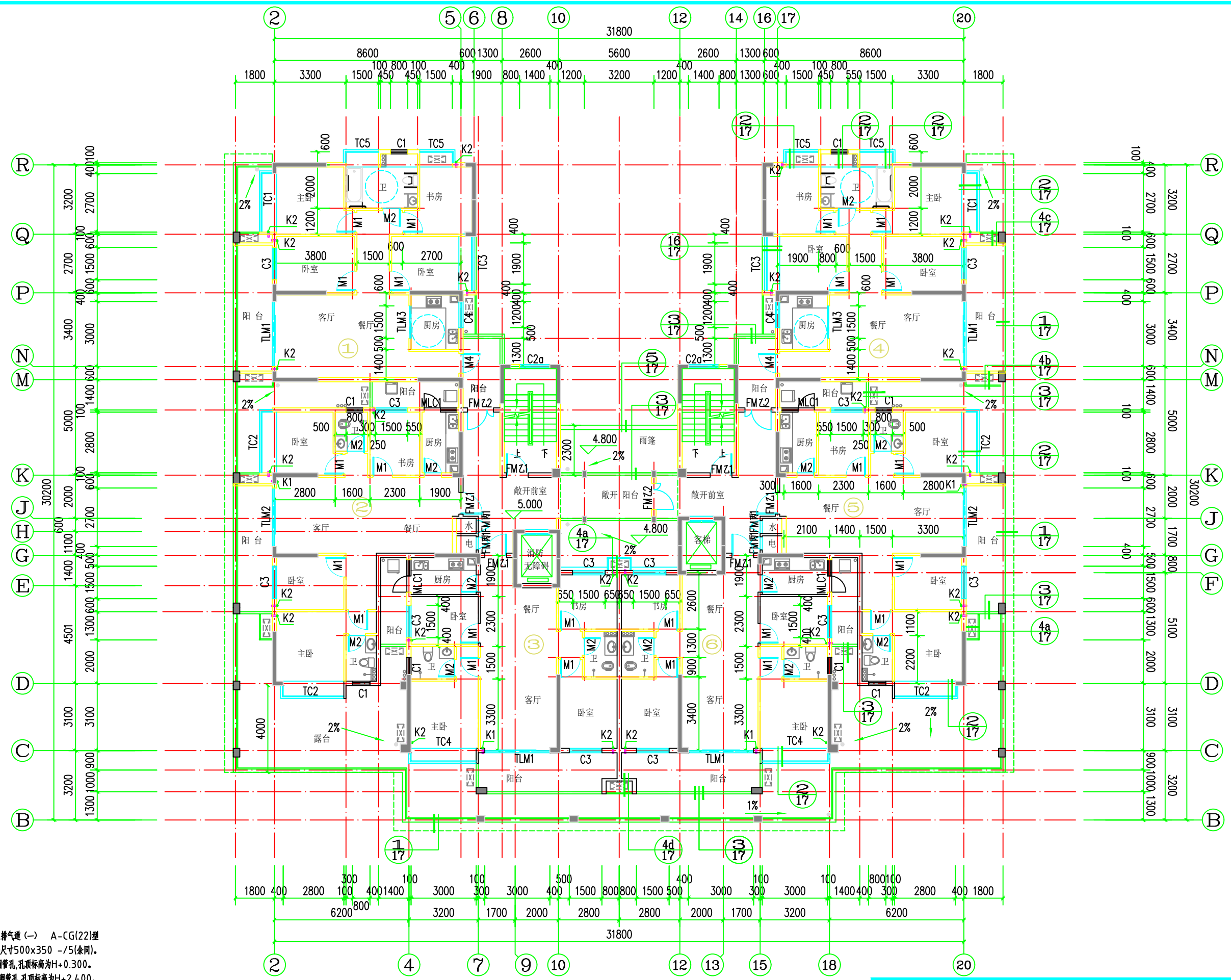
二层平面图 1:125 本层建筑面积: 671.73平方米
