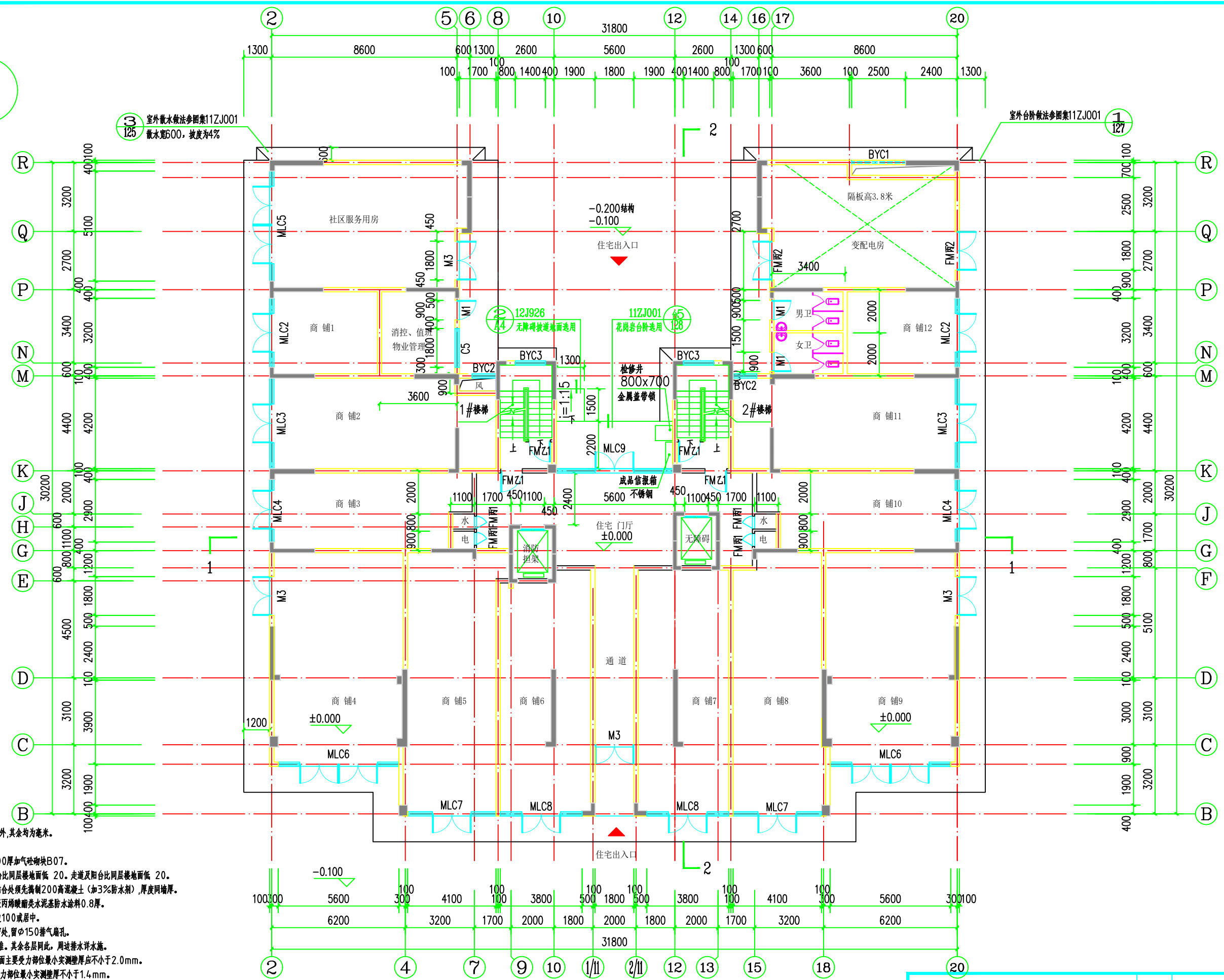
一层平面图 1:125 本层建筑面积: 797.25m 2
